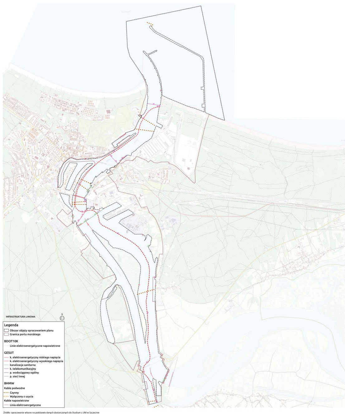
Ryc. 31. Lokalizacja liniowej infrastruktury technicznej na
