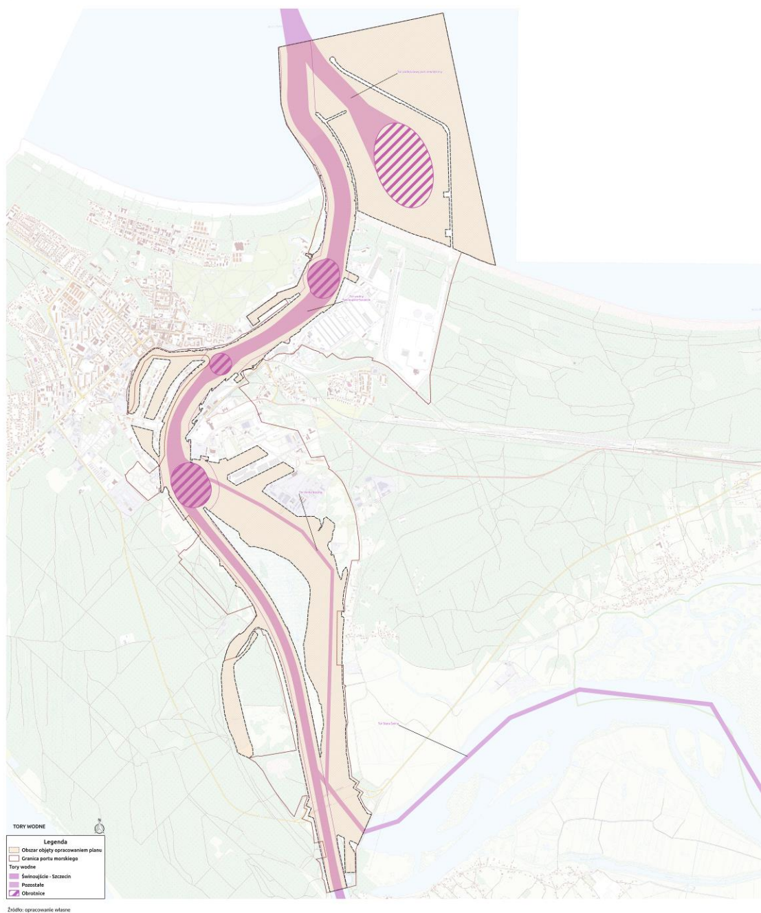
Ryc. 5. Lokalizacja torów wodnych na obszarze Portu
