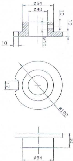
POZ.5 Skala 1:2.5
